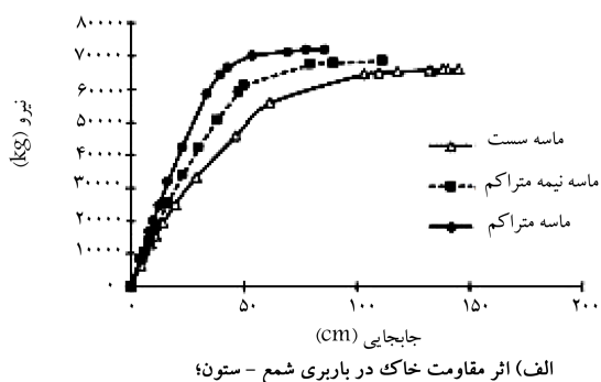
الف) اثر مقاومت خاک در باربری شمع - ستون؛
