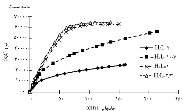
شکل ۸. ملاحظه‌ی مفهوم عمق بحرانی در دو ماسه‌ی متراکم و سست برای طول آزاد ۱۰ m.
