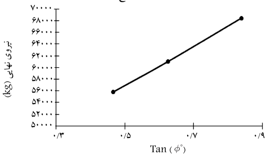
ب) مقاومت نهایی در برابر مقاومت خاک؛
