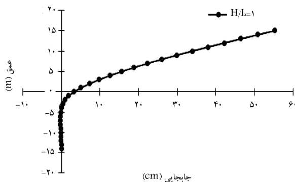
شکل ۶. رفتار شمع - ستون با طول مدفون ۱۵ متر در ماسه‌ی متراکم.
