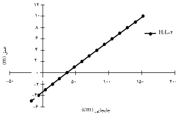
شکل ۷. رفتار شمع - ستون با طول مدفون ۵ متر در ماسه‌ی سُست.
