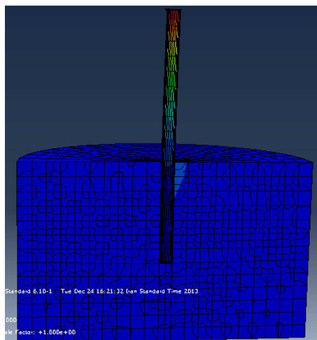
شکل ۳. تغییر شکل جانبی شمع در مدل عددی.
