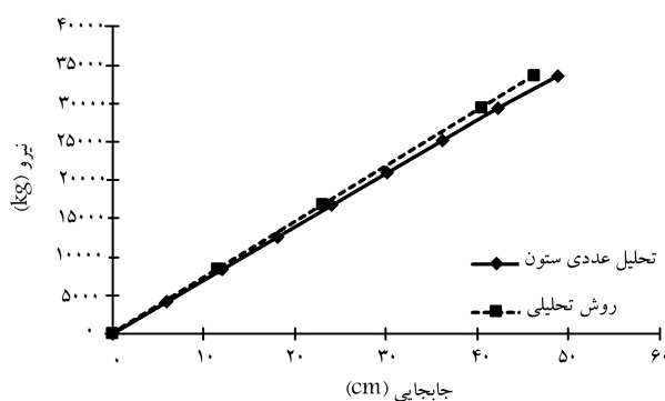
شکل ۴. مقایسه‌ی رفتار بار- جابه‌جایی جانبی حاصل از دو روش عددی و تحلیلی.
