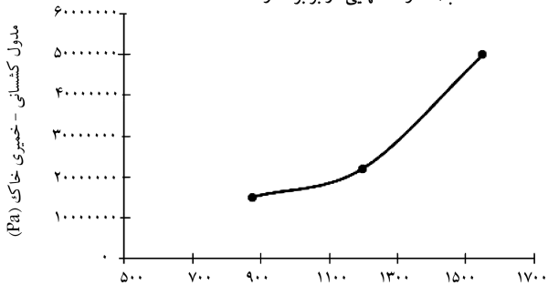
ج) سختی خمشی شمع ستون (kg/cm)
