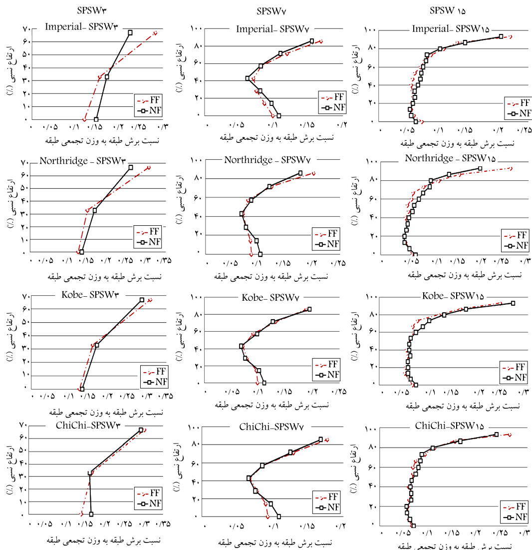
شکل ۵. نسبت بیشینه‌ی برش طبقه به وزن تجمعی سازه برای مدل‌های ۳، ۵ و ۷ طبقه.
