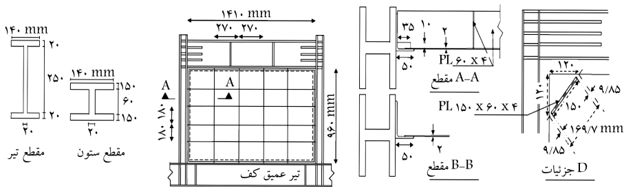
شکل ۲. مشخصات نمونه‌ی آزمایشگاهی دیوار برشی فولادی تقویت‌شده‌ی صبوری و سجادی. [۴]
