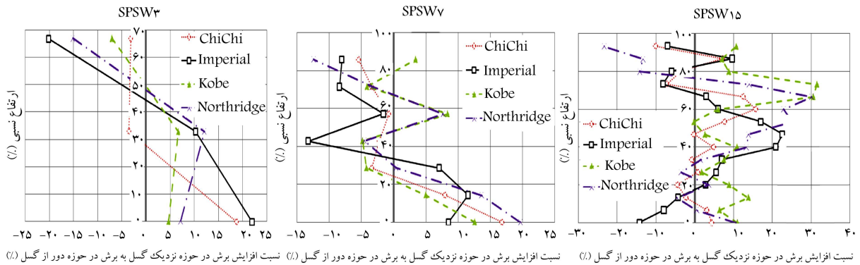
شکل ۶. نمودار افزایش نسبت برش پیش‌بینی نزدیک گسل به دور از گسل در برابر درصد ارتفاع مدل.
