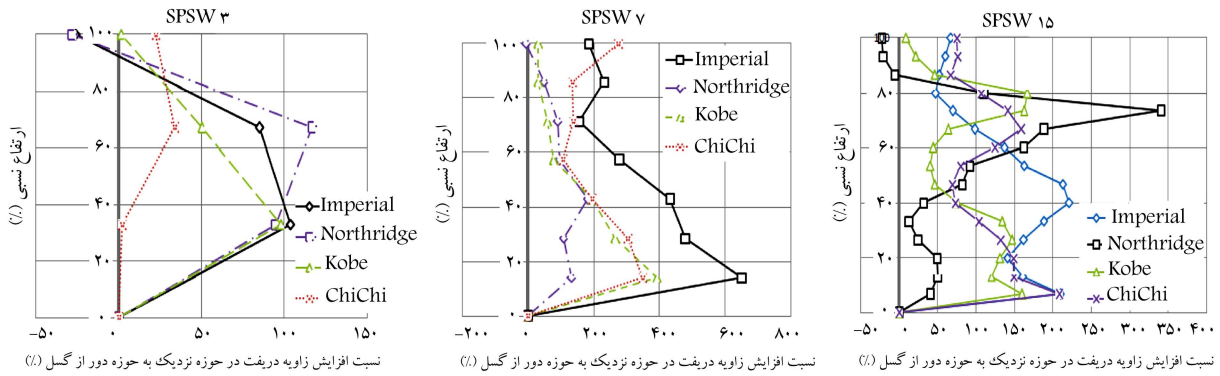
شکل ۸. نمودار درصد افزایش زاویه‌ی تغییرمکان نسبی طبقات در حوزی نزدیک گسل به حوزی دور از گسل.
