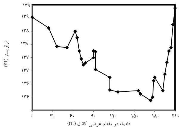
شکل ۶. مقطع عرضی اندازه‌گیری‌شده‌ی شماره‌ی ۹. [۸]
