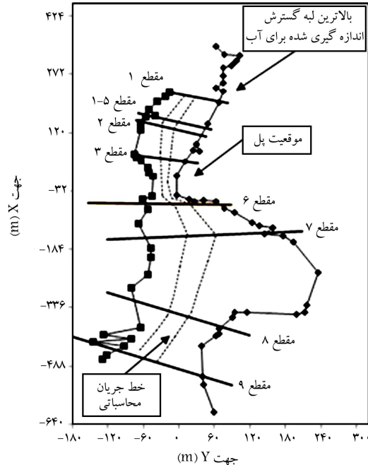
شکل ۵. پلان از محدوده‌ی مطالعاتی پل ۱۵ کالیفرنیا. [۸]
