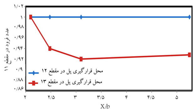
شکل ۱۱. تغییرات عدد فرود مقطع ۱۱ براساس نسبت‌های (x/b) متعدد در مقاطع در نظر گرفته شده برای احداث پل.
