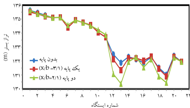
شکل ۱۲. تغییرات تراز بستر در مقاطع مختلف برای گام زمانی آخر براساس محاسبات نیمرخ برگشت آب.
