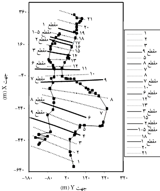
شکل ۴. پلان نشان‌دهنده‌ی موقعیت مقاطع عرضی به کار رفته در شبیه‌سازی عددی.
