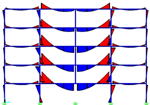
شکل ۱۴. لنگر خمشی اعضا بعد از حذف ستون.
