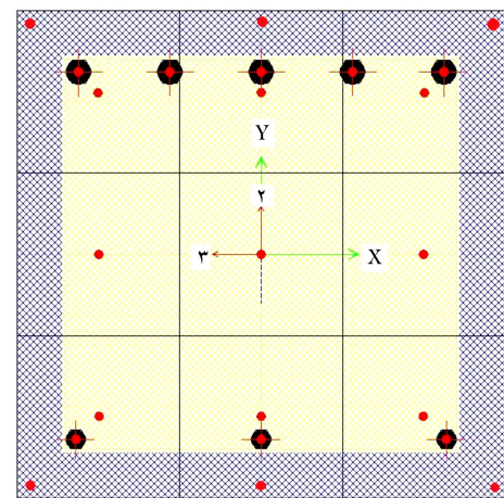
شکل ۲. محل قرارگیری فایبرها در مقطع تیرها.
