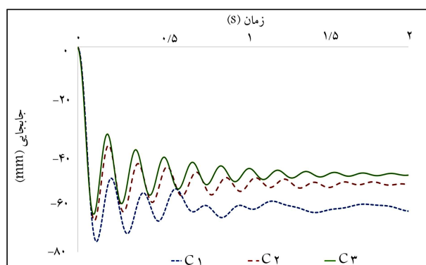
شکل ۱۶. جابه‌جایی بالای ستون‌های گوشه، کناری، و میانی برای شکل‌پذیری متوسط.
