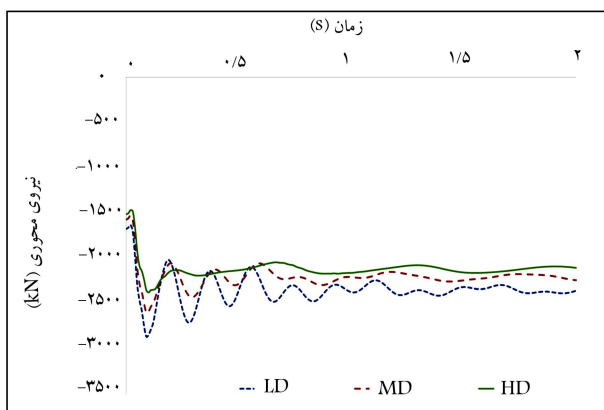
شکل ۶. تغییرات نیروی محوری ستون مجاور ستون حذف‌شده‌ی گوشه.
