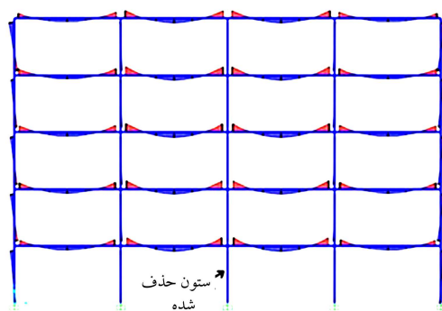
شکل ۱۳. لنگر خمشی اعضا قبل از حذف ستون.
