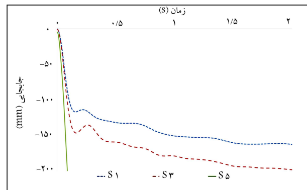
شکل ۲۰. جابه‌جایی قائم اتصال بالای ستون حذف‌شده‌ی گوشه برای شکل‌پذیری زیاد.
