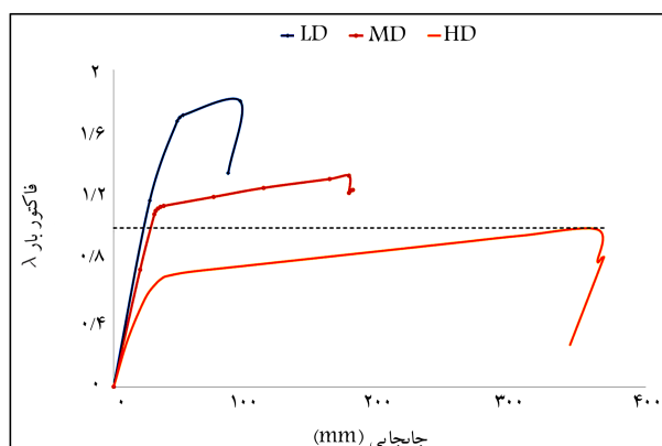
شکل ۴. پوش بار دهانه‌های بالای ستون حذف‌شده‌ی گوشه.
