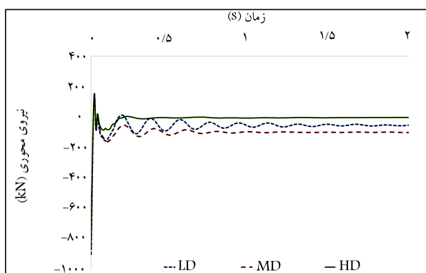
شکل ۷. تغییرات نیروی محوری ستون بالای ستون حذف‌شده‌ی گوشه.
