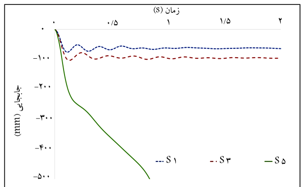
شکل ۱۹. جابه‌جایی قائم اتصال بالای ستون حذف‌شده‌ی گوشه برای شکل‌پذیری متوسط.
