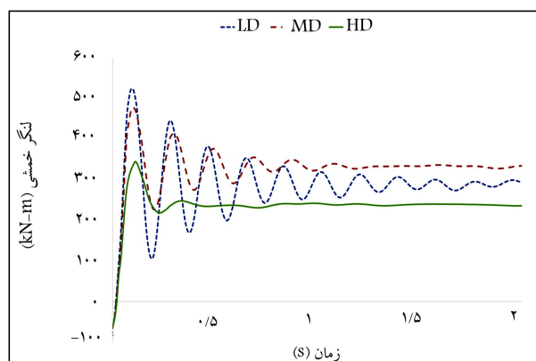
شکل ۵. تغییرات لنگر خمشی تیرهای متصل به ستون حذف‌شده‌ی گوشه.
