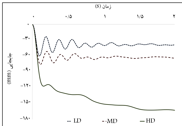
شکل ۳. جابه‌جایی بالای ستون حذف‌شده‌ی گوشه.
