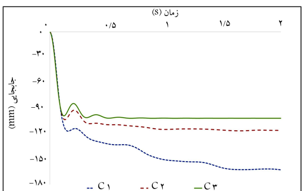
شکل ۱۷. جابه‌جایی گره بالایی ستون‌های حذف‌شده گوشه، کناری، و میانی برای شکل‌پذیری زیاد.
