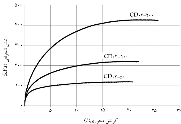
شکل ۱۱. نمودار \epsilon - q در آزمایش‌های زهکشی شده - گروه دوم ( R_c = \%87/11 ).
