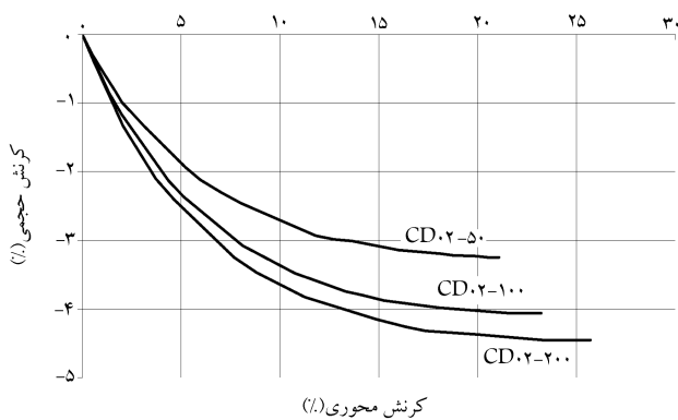
شکل ۱۲. نمودار \epsilon - \Delta \epsilon_v در آزمایش‌های زهکشی شده - گروه دوم ( R_c = \%87/11 ).
