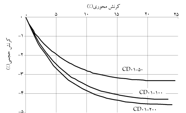
شکل ۱۰. نمودار \epsilon - \Delta \epsilon_v در آزمایش‌های زهکشی شده - گروه اول ( R_c = \%84/42 ).
