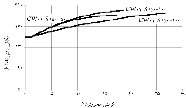
شکل ۲۰. نمودار تغییرات \epsilon - s در آزمایش‌های غیر اشباع - گروه اول - مکش بافتی اولیه ۱۵۰ کیلو پاسکال.
