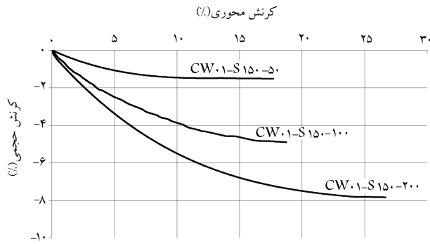
شکل ۱۹. نمودار تغییرات \epsilon - \epsilon_v در آزمایش‌های غیر اشباع - گروه اول - مکش بافتی اولیه ۱۵۰ کیلو پاسکال.
