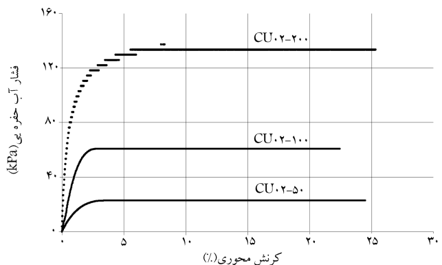
شکل ۸. نمودار \epsilon - \Delta u در آزمایش‌های زهکشی نشده - گروه دوم ( R_c = \%87/11 ).
