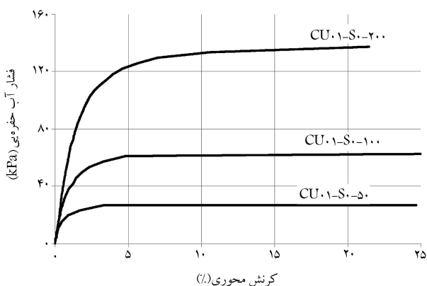
شکل ۶. نمودار \Delta u - \varepsilon در آزمایش‌های زهکشی نشده - گروه اول ( R_c = 84.42\% ).
