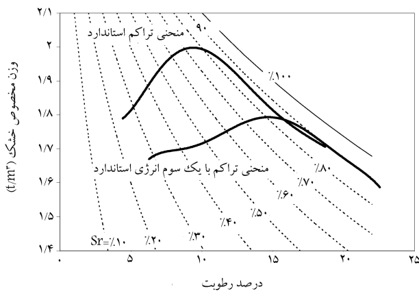
شکل ۴. منحنی‌های تراکم.
