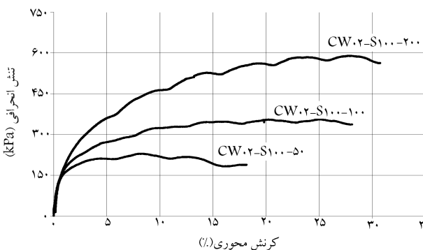
شکل ۲۴. نمودار تغییرات q - \varepsilon در آزمایش‌های غیراشباع - گروه دوم - مکش بافتی اولیه ۱۰۰ کیلو پاسکال.
