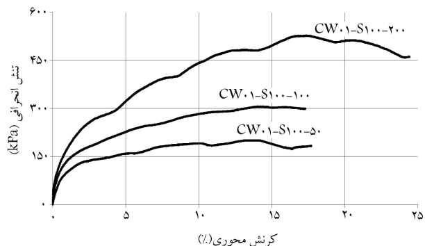
شکل ۲۱. نمودار تغییرات \epsilon - q در آزمایش‌های غیر اشباع - گروه اول - مکش بافتی اولیه ۱۰۰ کیلو پاسکال.
