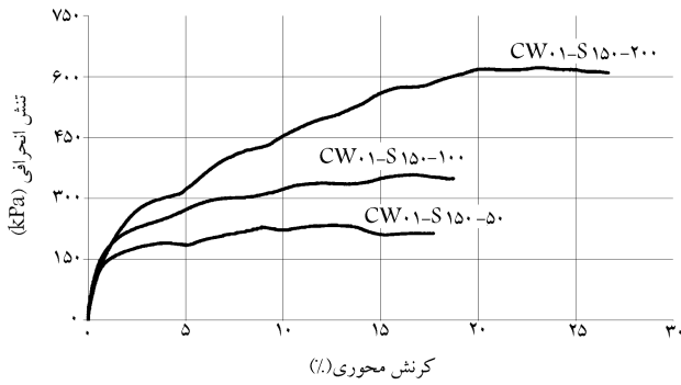
شکل ۱۸. نمودار تغییرات \epsilon - q در آزمایش‌های غیر اشباع - گروه اول - مکش بافتی اولیه ۱۵۰ کیلو پاسکال.
