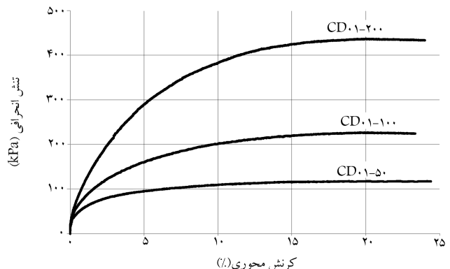
شکل ۹. نمودار \epsilon - q در آزمایش‌های زهکشی شده - گروه اول ( R_c = \%84/42 ).
