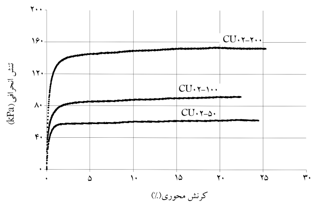
شکل ۷. نمودار \epsilon - q در آزمایش‌های زهکشی نشده - گروه دوم ( R_c = \%87/11 ).
