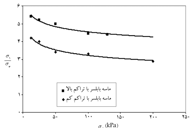
شکل ۴. تغییرات نسبت \frac{\sigma_1}{\sigma_3} در برابر \sigma_3 برای ماسه‌ی بابلسر در دو نمونه با چگالی نسبی ۰/۱۳/۳ و ۰/۹۰.
