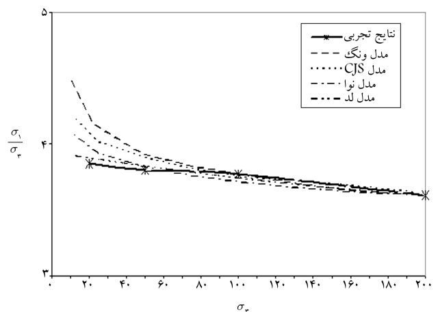
شکل ۹. تغییرات نسبت \frac{\sigma_1}{\sigma_3} در برابر \sigma_3 برای ماسه‌ی تویورا با تراکم کم.
