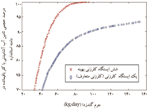
شکل ۴. رویه‌های بهینه‌ی پارتوکل کلر مصرفی و درصد حجمی تامین آب آشامیدنی با کلر باقیمانده در دامنه‌ی استاندارد.
