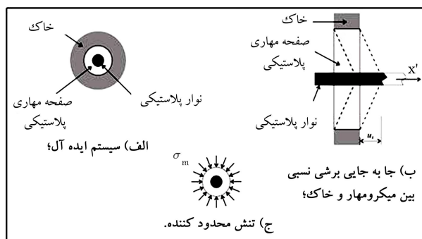
شکل ۴. رفتار و هندسه‌ی مهار - شبکه‌ها به‌عنوان المان مسلح‌کننده در مدل‌سازی عددی. [۱۷]
