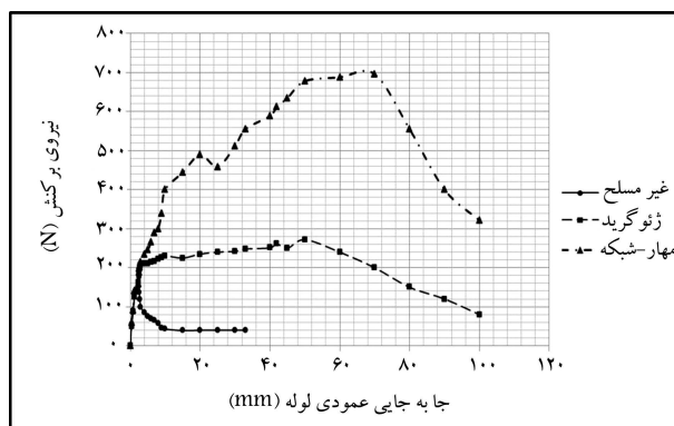
شکل ۶. تغییرات مقاومت برکنش بیشینه در برابر جابه‌جایی عمودی لوله در ماسه‌ی خشک حاصل از مطالعات آزمایشگاهی ( b = 5D , h/D = 2 , N = 1 , D = 50 \text{ mm} )
