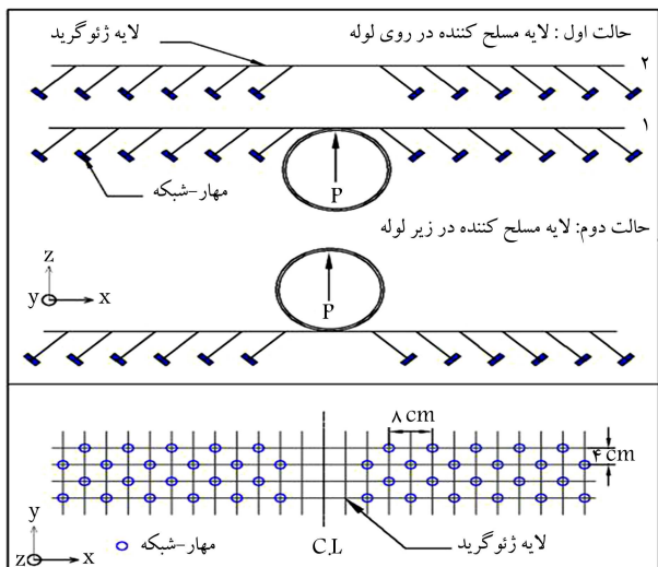
شکل ۱. نحوه‌ی به‌کارگیری سیستم مهار - شبکه به‌طور شماتیک.
