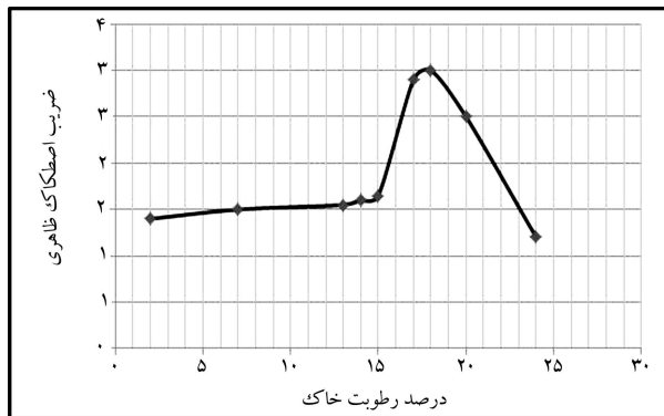
شکل ۱۲. تغییر ضریب زاویه اصطکاک ظاهری خاک با افزایش میزان رطوبت آن. [۱۹]
