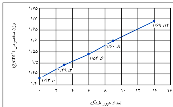
شکل ۳. تغییرات وزن مخصوص به تعداد عبور غلتک برای رسیدن به چگالی مورد نظر. [۲۲]
