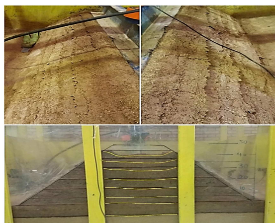
شکل ۲۰. نشست ها و سطوح گسیختگی در خاکریز ELM2.
