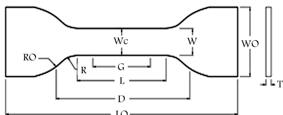
شکل ۹. شماتیک نمونه‌ی آزمایش کشش.
