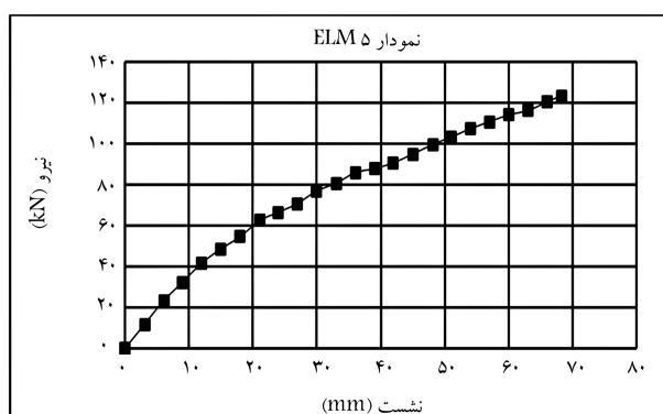
شکل ۲۵. نمودار نیرو - جابه‌جایی برای خاکریز ELM۵.
