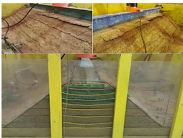
شکل ۲۶. نشست‌ها و سطوح گسیختگی در خاکریز ELM۵.
