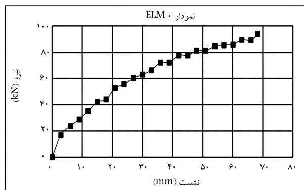
شکل ۱۴. نمودار نیرو - جابه‌جایی برای خاکریز ELM^0 .
