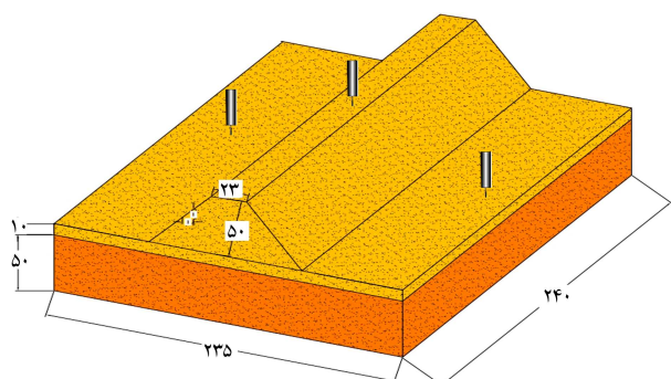
شکل ۱۱. خاکریز و ابعاد آن به سانتی‌متر. [۲۱]
