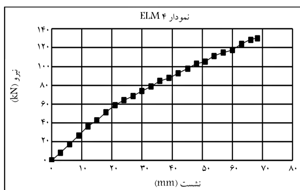
شکل ۲۳. نمودار نیرو - جابه‌جایی برای خاکریز ELM۴.
