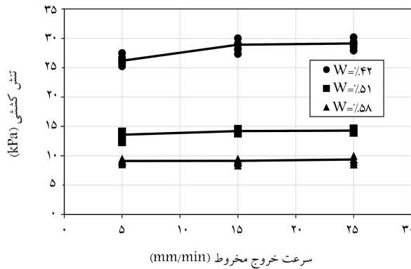
شکل ۴. نمودار تغییر سرعت جدایش مخروط در برابر تنش کششی برای نمونه‌ی S۱ در درصد رطوبت‌های مختلف.
