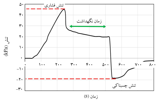
شکل ۳. نمودار تنش فشاری و کششی در مقابل زمان برای رطوبت ۵۰٪ مربوط به نمونه‌ی S۲.
