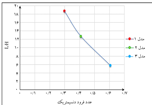
شکل ۹. نمودار نسبت طول نفوذ شوری به تراز رودخانه به عدد فرود دنسیمیتریک.
