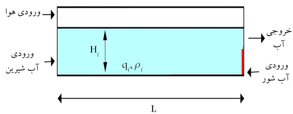
شکل ۱. هندسه‌ی مدل.
