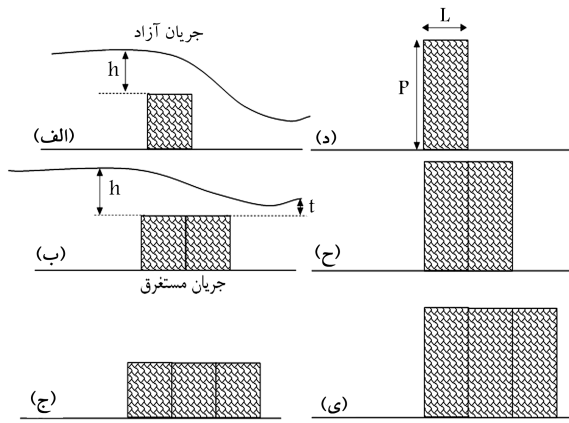
شکل ۱. شمای سرریز لبه پهن گابیونی.
