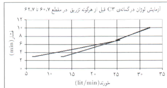
شکل ۱۲. نمودار فشار آزمایش و مقدار جذب آب در گمانه‌ی C۳ قبل از تزریق. [۱۸]
