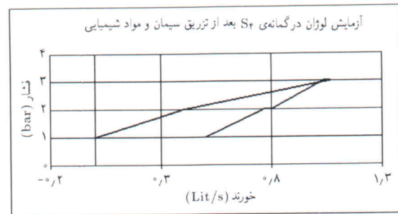
شکل ۹. نمودار فشار آزمایش و مقدار آب در گمانه‌ی S4 بعد از تزریق سیمان و مواد شیمیایی. [۱۷]
