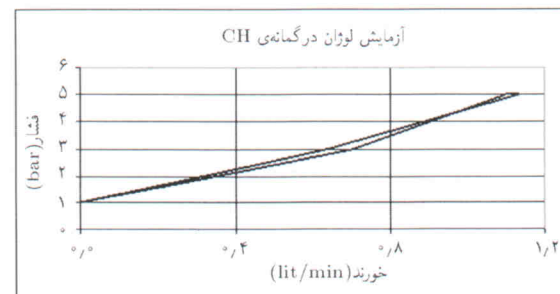
شکل ۱۳. نمودار فشار آزمایش و مقدار جذب آب در گمانه‌ی CH بعد از تزریق. [۱۸]
