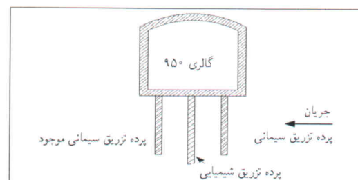
شکل ۱۴. مقطع گالری ۹۵° با تزریق ساندویچی.
