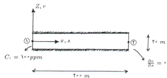
شکل ۹. نمای مسئله در مثال ۱.
