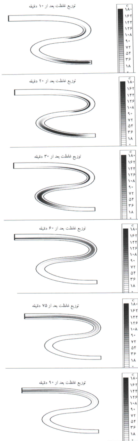
شکل ۱۱. تغییرات توزیع آلودگی با زمان در مثال ۲.
