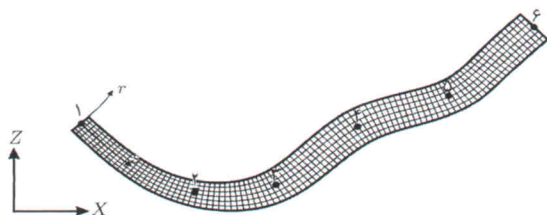
شکل ۳. شبکه‌بندی رودخانه.
