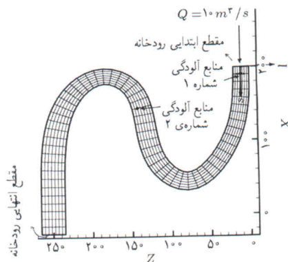
شکل ۹. نمای رودخانه و شبکه‌بندی در مسئله ۲.
