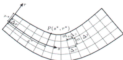
شکل ۱. دستگاه مختصات (s, r) منحنی الخط.
