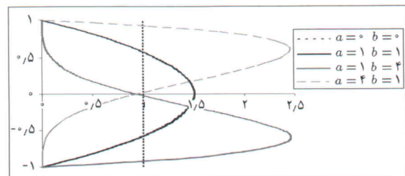
شکل ۴. توزیع سرعت به ازای a و b های مختلف.
