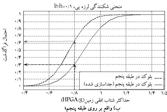
شکل ۱۵. مقایسه‌ی منحنی‌های شکنندگی برای بلوک‌های صلب، با نسبت ابعاد b/h = 0.1 خط پر: کف جداسازی شده، نقطه چین: جداسازی نشد.
