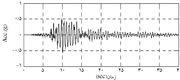
و) تاریخچه زمانی شتاب طبقه 4 تحت زلزله ال سنتر و PGA=0.3
