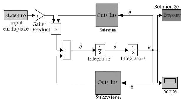
شکل ۳. نمودار محاسبه تاریخچه‌ی زمانی پاسخ دوران بلوک تحت اثر زلزله، در MATLAB و SIMULINK.
