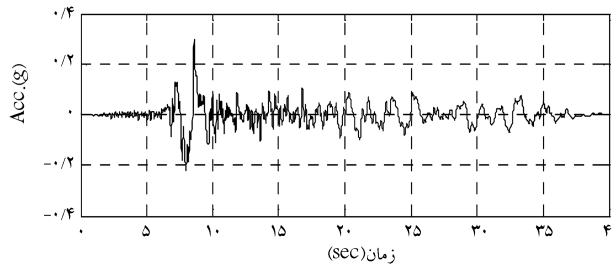
ه) تاریخچه زمانی شتاب زلزله ال سنتر و PGA=0.3
