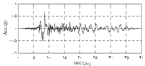
الف) تاریخچه زمانی شتاب زلزله ال سنتر و PGA=0.7
