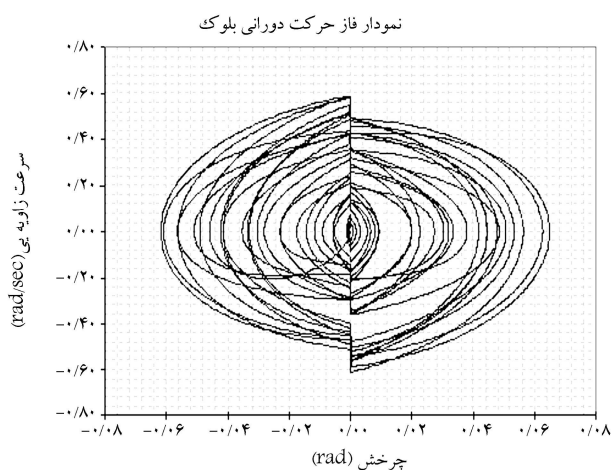
ب) نمودار سرعت زاویه‌ی بلوک بر حسب دوران بلوک (Phase Plot) ( b/h=0.75 )
