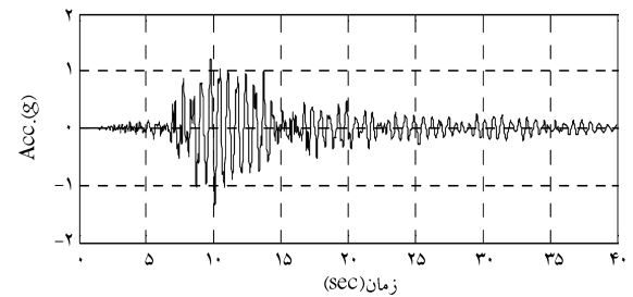
ب) تاریخچه زمانی شتاب طبقه 4 تحت زلزله ال سنتر و PGA=0.7
