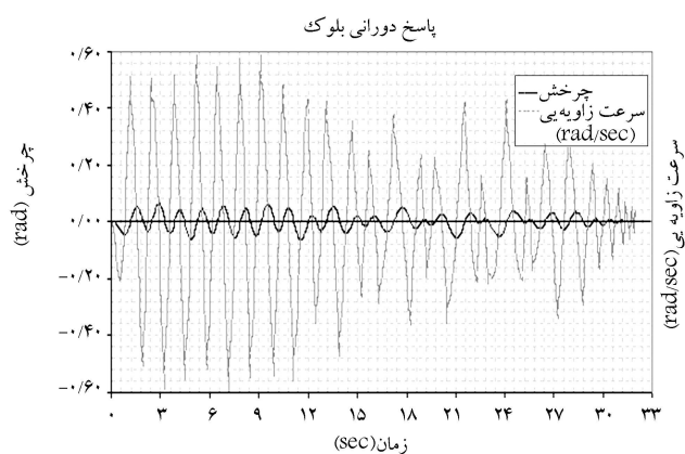
الف) تاریخچه‌ی زمانی پاسخ دوران و سرعت زاویه‌ی بلوک تحت زلزله ال-سنترو؛
