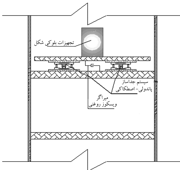
الف) نمای شماتیک از کف جلدسازی شده در طبقات ساختمان؛
