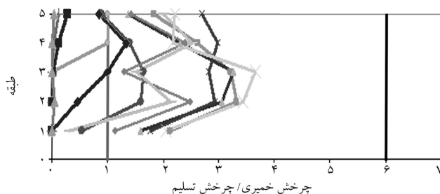
چرخش خمیری / چرخش تسلیم
