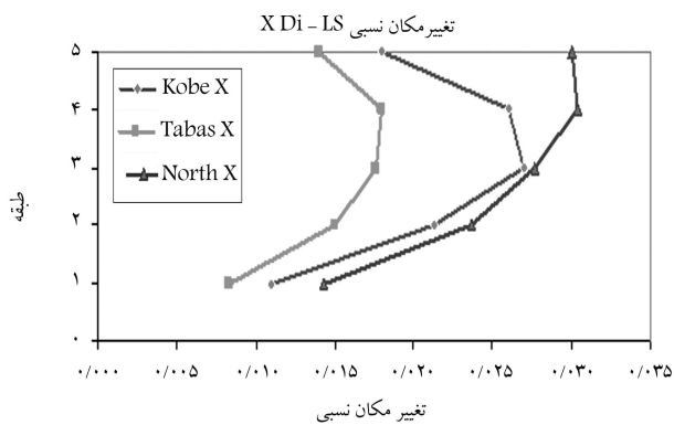
شکل ۵. بیشینه نسبت تغییر مکان درون طبقه‌ی در سازه‌ی ۵ طبقه‌ی صلب، در راستای x و y.
