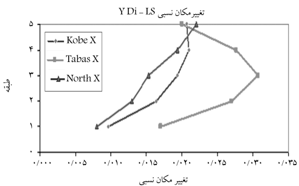
شکل ۶. بیشینه نسبت تغییر مکان درون طبقه‌ی در سازه‌ی ۵ طبقه‌ی نرم، در راستای x و y.
