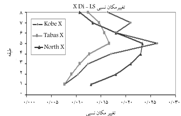
شکل ۷. بیشینه نسبت تغییر مکان درون طبقه‌ی در سازه‌ی ۸ طبقه‌ی صلب، در راستای x و y.
