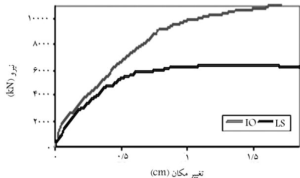
ب) ۸ طبقه در دو حالت سطح عملکرد متعارف و کاهش یافته در تحلیل بارافزون.
