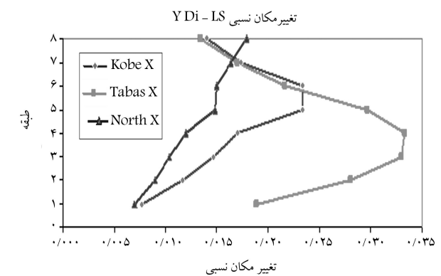
شکل ۸. بیشینه نسبت تغییر مکان درون طبقه‌ی در سازه‌ی ۸ طبقه‌ی نرم، در راستای x و y.
