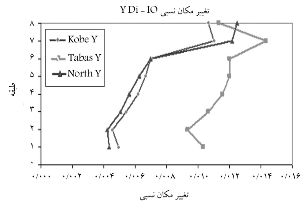
شکل ۷. بیشینه نسبت تغییر مکان درون طبقه‌ی در سازه‌ی ۸ طبقه‌ی صلب، در راستای x و y.
