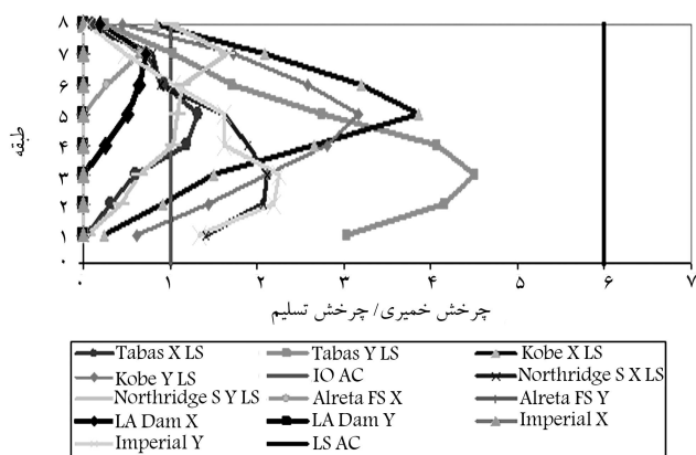
ب) نرم در برابر جنبش های نزدیک به گسل.
