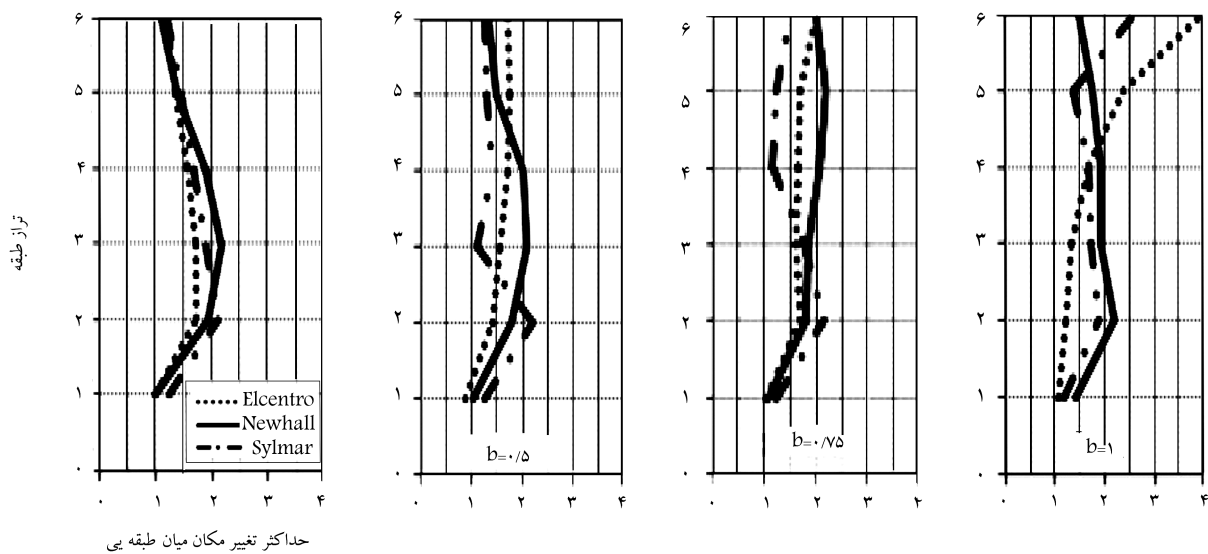
شکل ۲. بیشترین تغییر مکان جانبی نسبی ۴ قاب ۶ طبقه‌ی مهاربندی شده‌ی واگرای خمشی برای مقادیر متفاوت b .
