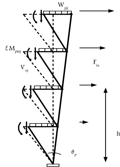
شکل ۶. نمودار آزاد ستون مشترک دهانه‌های s و s-1 در قاب شکل ۱، در وضعیت تغییرشکل یافته‌ی نهایی.
