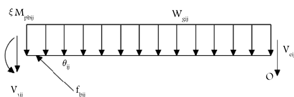
شکل ۵. نمودار آزاد تیر خارج از تیر پیوند در قاب مهاربندی واگرا.
