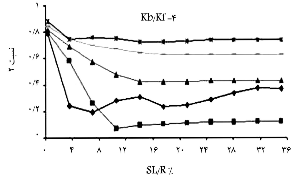
شکل ۷. نمودار بار لغزشی بهینه برای تعادل پیچشی قوی و ضعیف برای مدل‌های ۱-۵ به ازای نسبت سختی مهاربند به قاب ۲، ۳ و ۴.
