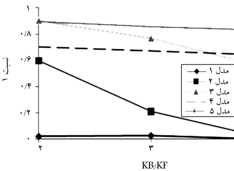
شکل ۸. نمودار نسبت سختی مهاربند به قاب بهینه برای تعادل پیچشی قوی و ضعیف برای مدل‌های ۱-۵.
