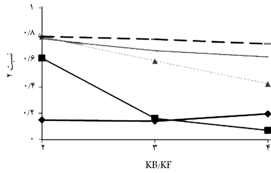
شکل ۸. نمودار نسبت سختی مهاربند به قاب بهینه برای تعادل پیچشی قوی و ضعیف برای مدل‌های ۱-۵.
