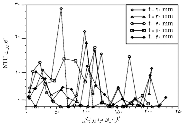
شکل ۴. نتایج آزمایشگاهی کدورت نسبت به گرادیان هیدرولیکی (t ضخامت فیلتر). [۱۱]
