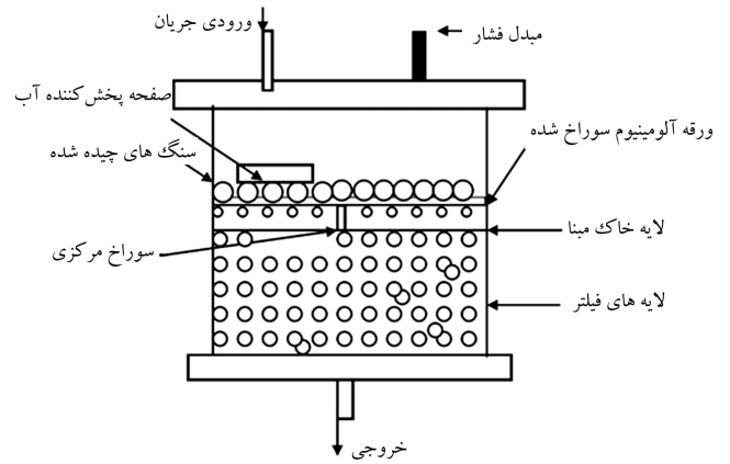
شکل ۳. دستگاه استفاده شده برای تعیین گرادیان هیدرولیکی بحرانی. [۱۱]
