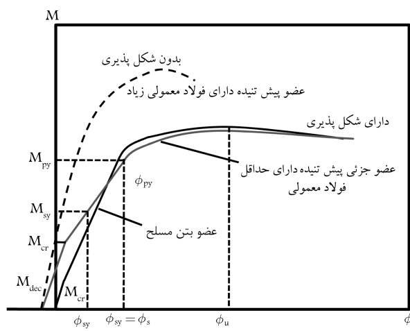
الف) منحنی ممان - انحنای [۹]
