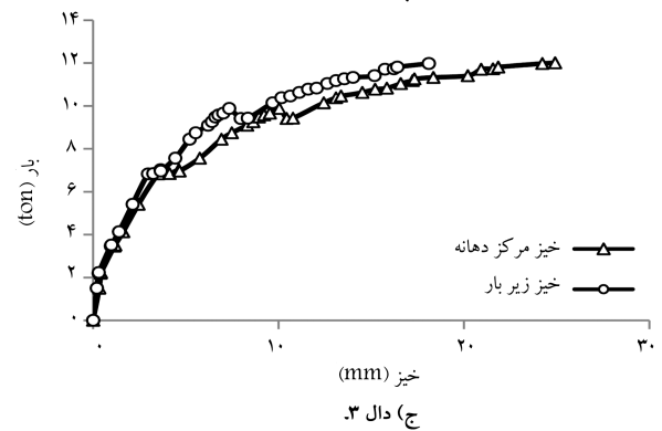
شکل ۸. نمودار بار-خیز.
