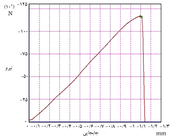
شکل ۵. منحنی بار - جابجایی یکی از نمونه‌های آزمون‌شده آسفالت.
