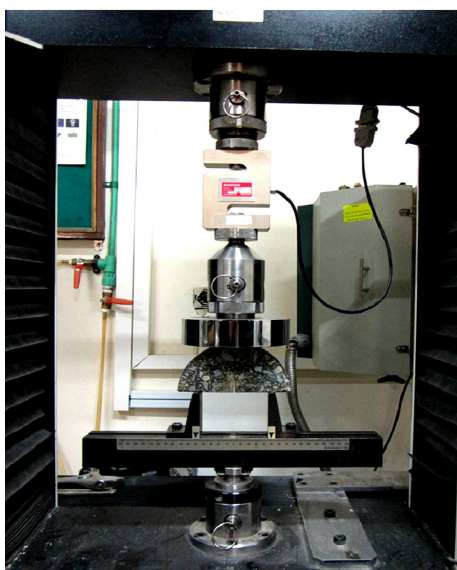
شکل ۴. نمای از نحوه‌ی بارگذاری.
