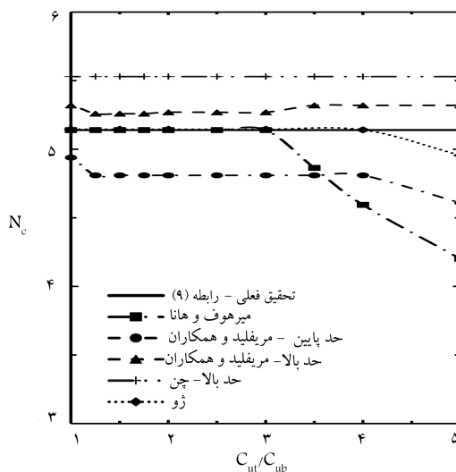
شکل ۱۵. تغییرات ضریب ظرفیت باربری در حالت خاک سخت روی خاک نرم برای H/B = 2 .
