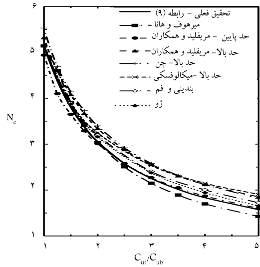
شکل ۱۱. تغییرات ضریب ظرفیت باربری در حالت خاک سخت روی خاک نرم برای H/B = ۰٫۲۵ .
