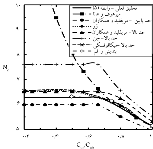
شکل ۸. تغییرات ضریب ظرفیت باربری در حالت خاک نرم روی خاک سخت برای H/B = 0.25
