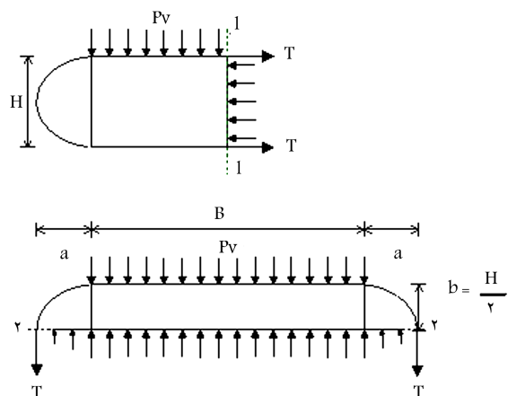
ب) سیستم کیسه - خاک تحت فشار P_V و کشش T در برش‌های ۱-۱ و ۲-۲.
