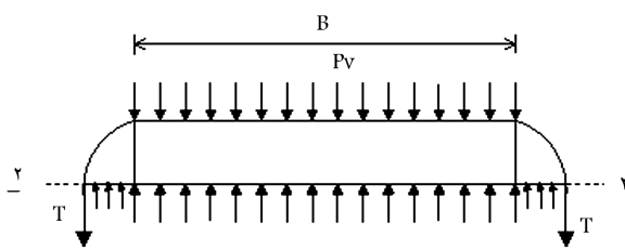
ب) سیستم کیسه - خاک تحت فشار P_v و کشش T در برش های ۱-۱ و ۲-۲.
