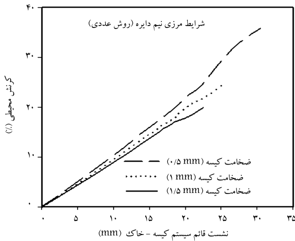
شکل ۱۳. جابجایی قائم سیستم کیسه - خاک به کرنش محیطی کیسه.
