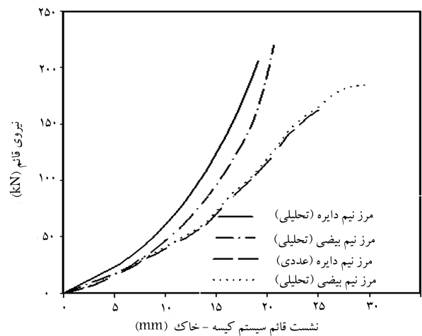
شکل ۱۱. تغییرات جابجایی سیستم کیسه - خاک به بارگذاری قائم.
