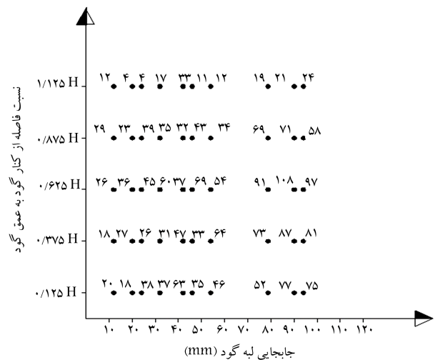
شکل ۱۰. مقادیر DPI به‌ازاء مقادیر مختلف جابجایی تاج و فاصله از بر گود.
