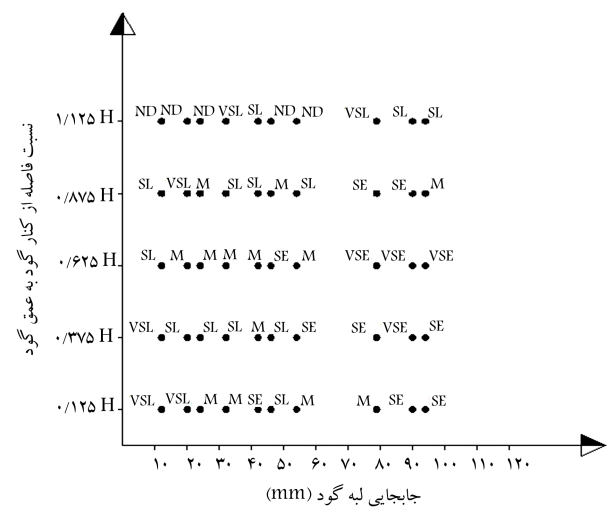
شکل ۱۱. درجات خرابی سازه‌ی مجاور گود به‌ازاء مقادیر مختلف جابجایی تاج و فاصله از بر گود مطابق با تعریف جدول ۲.
