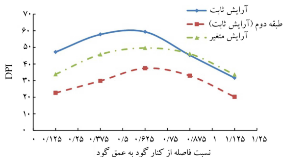
شکل ۶. مقادیر درجه‌ی خرابی در ۲ طبقه‌ی سازه و در ۲ آرایش میخ‌کوبی با طول ثابت و طول متغیر.
