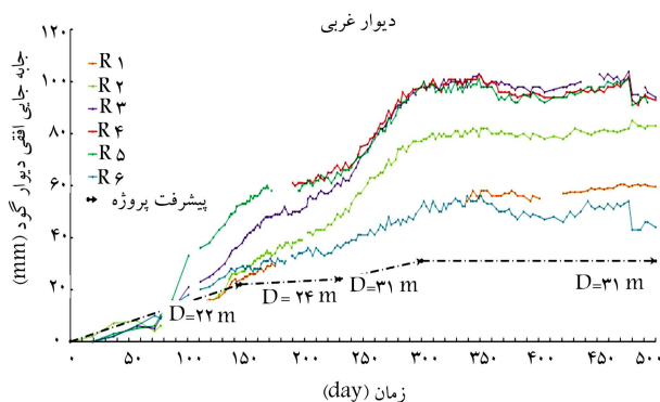
شکل ۷. نمونه‌ی نتایج مانتیورینگ دیواره‌ی میخ‌کوبی شده.
