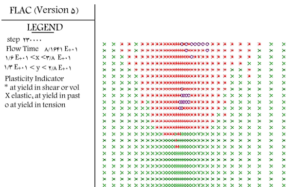
شکل ۱۵. به تسلیم رسیدن در زمان وقوع جوشش.
