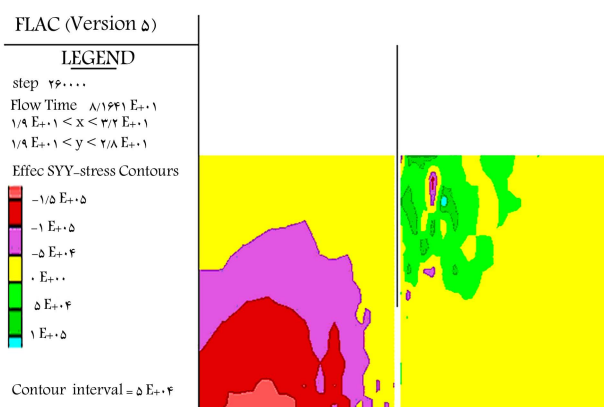
شکل ۱۶. تنش مؤثر زمان وقوع جوشش به ازاء عمق پردی آب‌بند ۳۰ cm.
