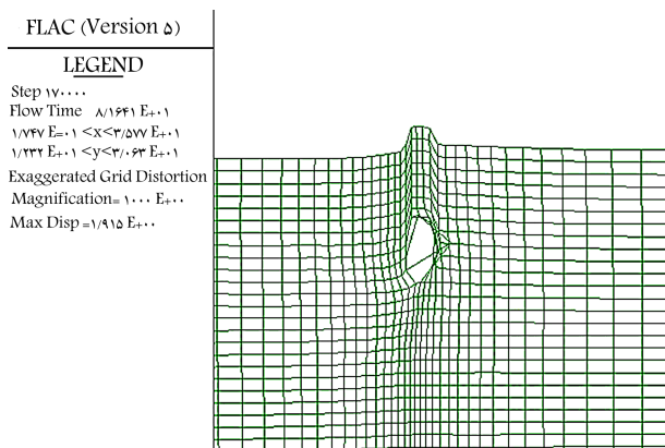
شکل ۱۹. تغییر شکل در زمان وقوع بالازدگی منشور مستطیلی.
