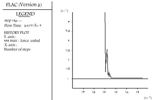
شکل ۹. نمودار پیشینه‌ی نیروی نامتعادل در زمان وقوع جوشش به ازاء عمق پرده‌ی آببند 30 سانتی‌متر.
