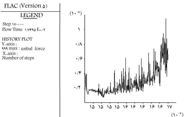
شکل ۱۳. نیروی نامتعادل در زمان وقوع جوشش.
