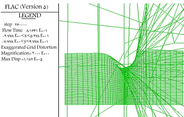
شکل ۱۴. تغییر شکل در زمان وقوع جوشش.
