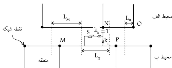
شکل ۶. مدل‌سازی اتصال دو المان متفاوت در FLAC. [۱۲]
