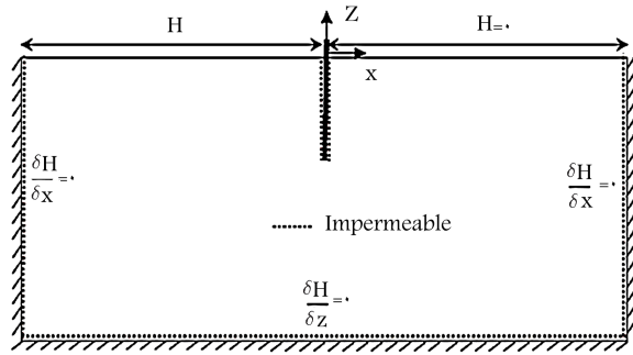
شکل ۱۱. شرایط مرزی هیدرولیکی.
