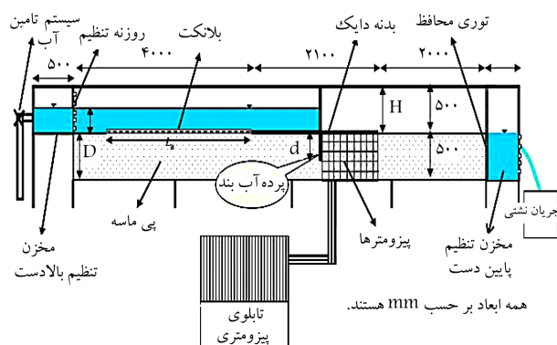
شکل ۷. شماتیک مدل آزمایشگاهی. [۱۰]
