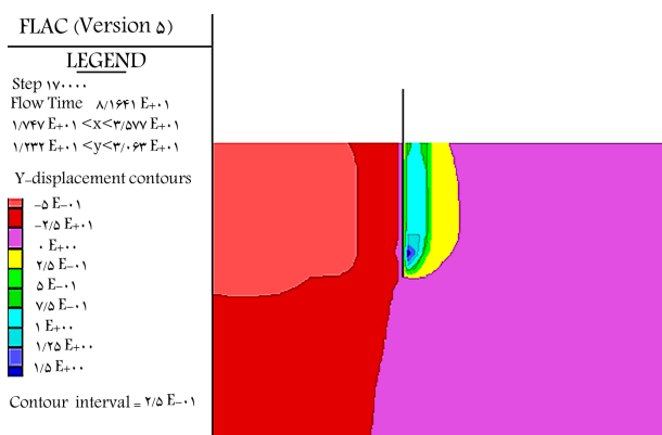
شکل ۱۸. جابه‌جایی در جهت y زمان وقوع بالازدگی منشور مستطیلی.
