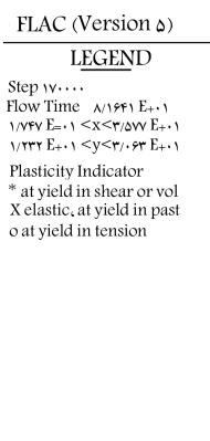
شکل ۲۵. به تسلیم رسیدن در زمان وقوع بالازدگی منشور مستطیلی.
