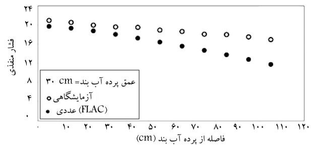
شکل ۸. چگونگی کاهش فشار بالاتر در عمق پرده‌ی آببند 30 سانتی‌متر.
