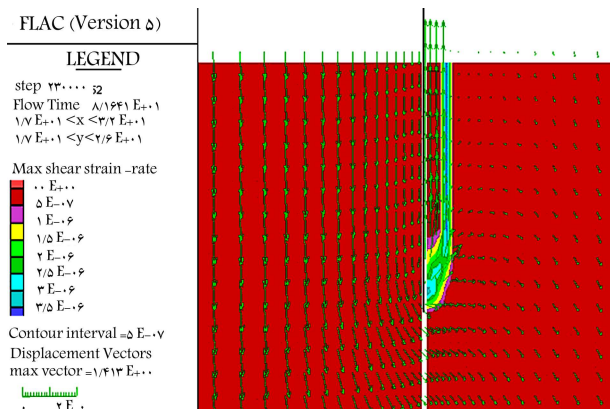
شکل ۱۷. نرخ کرنش در زمان وقوع بالازدگی منشور مستطیلی.
