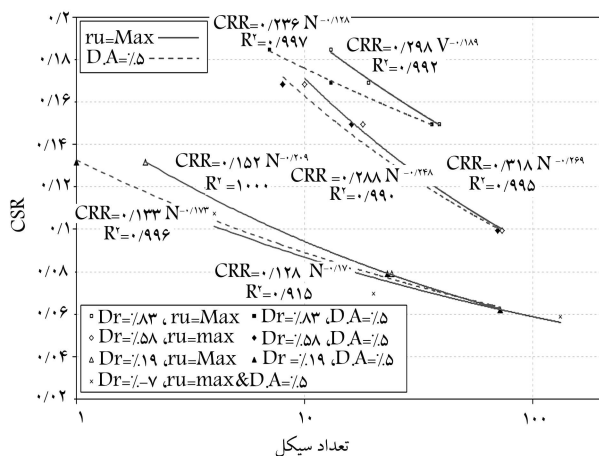
شکل ۶. مقاومت روان‌گرایی ماسه‌ی فیروزکوه در برابر تعداد سیکل در تراکم‌های مختلف.
