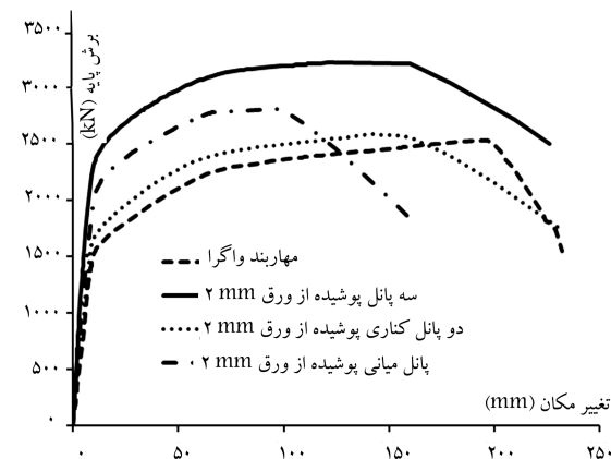
شکل ۱۴. نمودار بار - تغییر مکان سیستم‌های ترکیبی و مهاربند واگرا برای ورق‌های با ضخامت مختلف.
