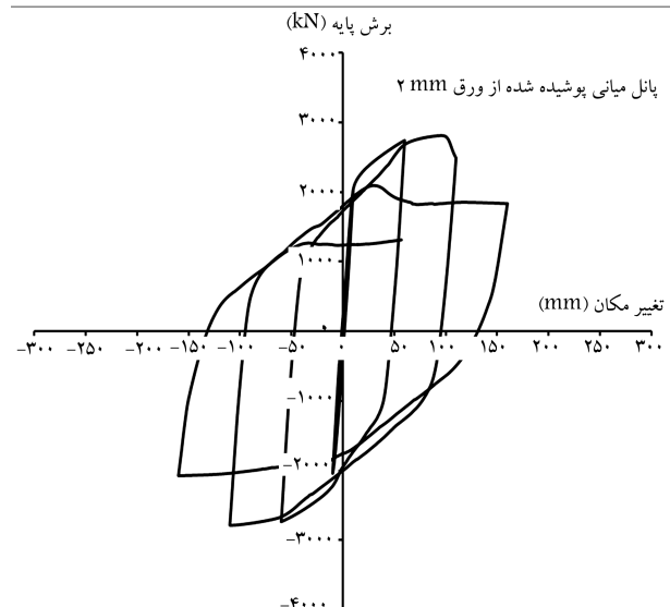
شکل ۱۶. رفتار هیستریزیس سیستم ترکیبی با ورق پُرکننده‌ی ۲ میلی‌متری.
