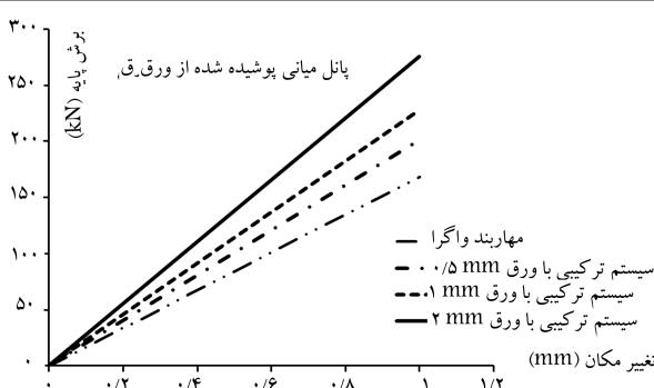
شکل ۱۱. تأثیر ورق‌های نازک پُرکننده بر سختی مهاربند و اگر.
