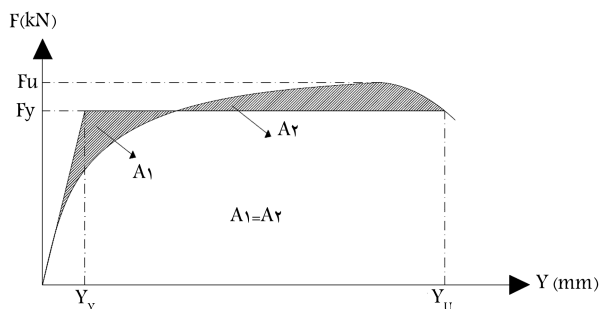
شکل ۱۲. نمودار بار تغییرمکان واقعی و ایده آل سازه.
