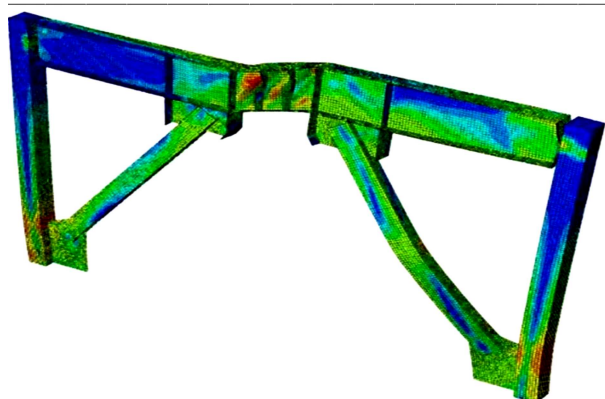
شکل ۱۳. رفتار چرخه‌ای و تغییرشکل قاب مهاربند واگرا.
