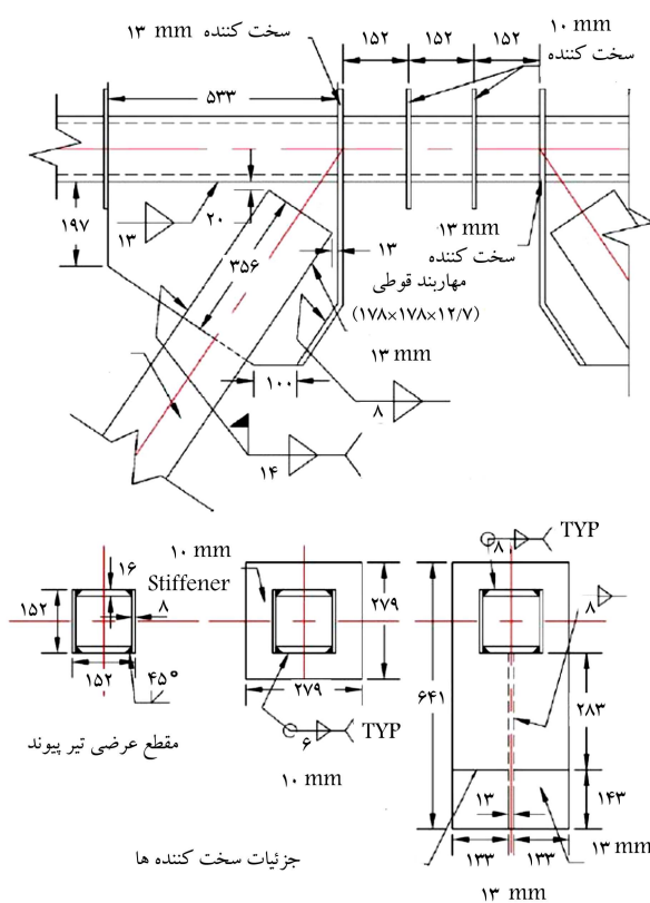
شکل ۳. جزئیات مدل آزمایشگاهی مهاربند واگرا. [۱۳]
