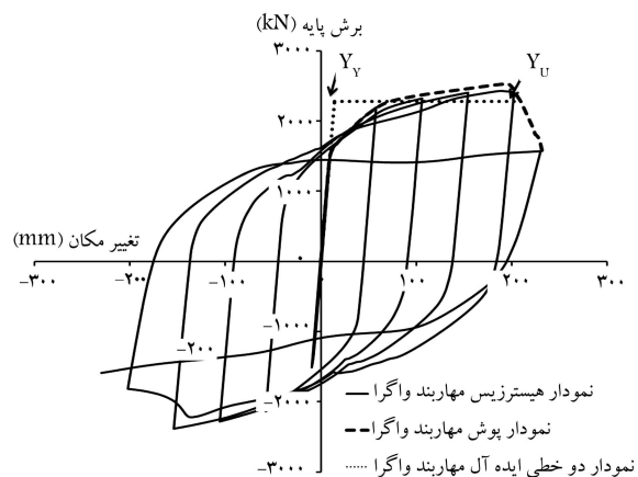
شکل ۱۲. نمودار بار تغییرمکان واقعی و ایده آل سازه.
