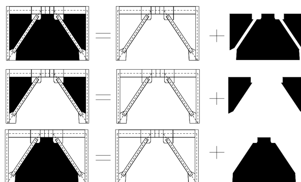
شکل ۹. جمع‌پذیری ورق‌های فولادی و مهاربند واگرا.
