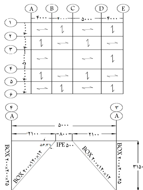
شکل ۱. ابعاد پلان ساختمان و قاب مهاربندی طبقه‌ی اول (بر حسب میلی‌متر).
