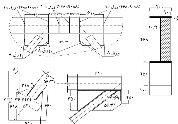
شکل ۲. جزئیات اجرایی اتصالات قاب مهاربندی (بر حسب میلی‌متر).
