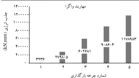
شکل ۱۵. منحنی هیستریزیس و میزان جذب انرژی مهاربند واگرا.
